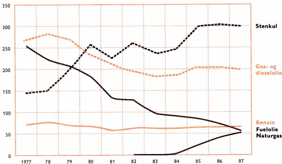
Bruttoenergiforbruget for stenkul, fuelolie, gas- og dieselolie, benzin og naturgas
